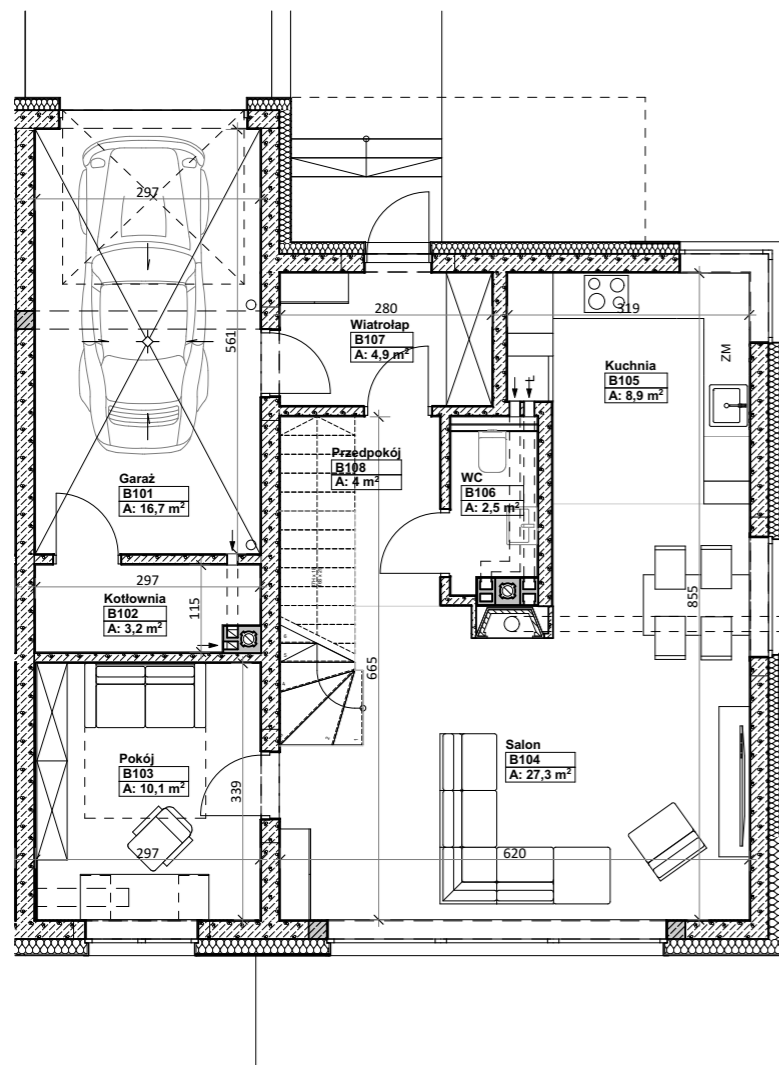
RZUT PARTERU
